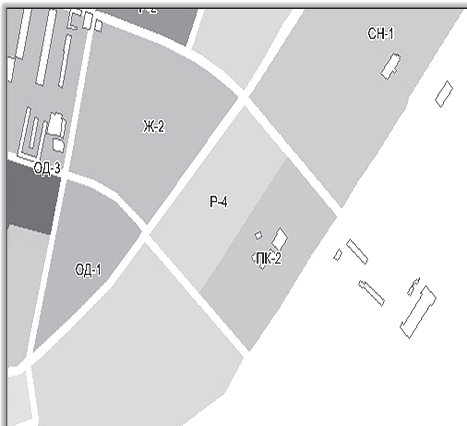
Фрагмент карты градостроительного зонирования в районе ул. Железнодорожная, 115 до внесения изменений в правила землепользования и застройки
