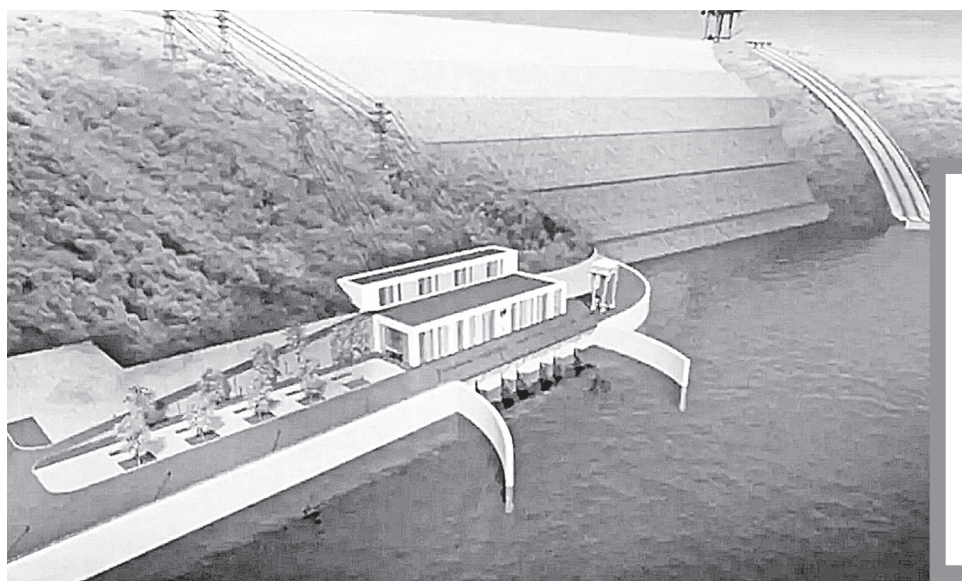
Нижне-Ниманская ГЭС (схема)
