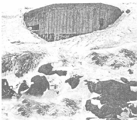
Долговременная огневая точка - ДОТ. Меньшиково, 2004 год
